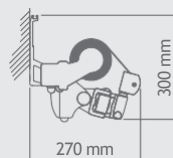
Montāža pie sienas
