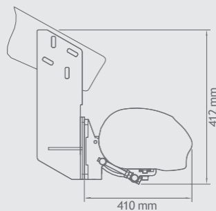
Montāža pie slīpa jumta
