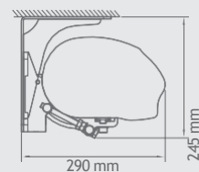
Montāža pie jumta kores
