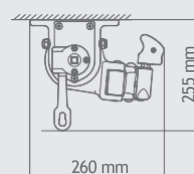
Montāža pie jumta kores
