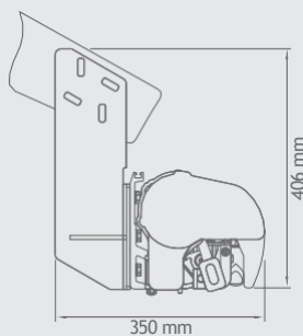
Montāža slīpā jumtā
