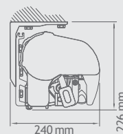
Montāža pie jumta kores
